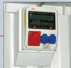
Verteilerkasten mit integrierten Steckdosen
